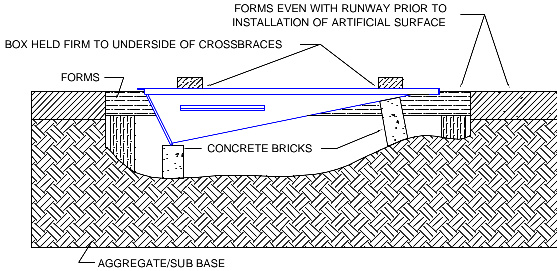
SIDE VIEW PRIOR TO CONCRETE POUR
