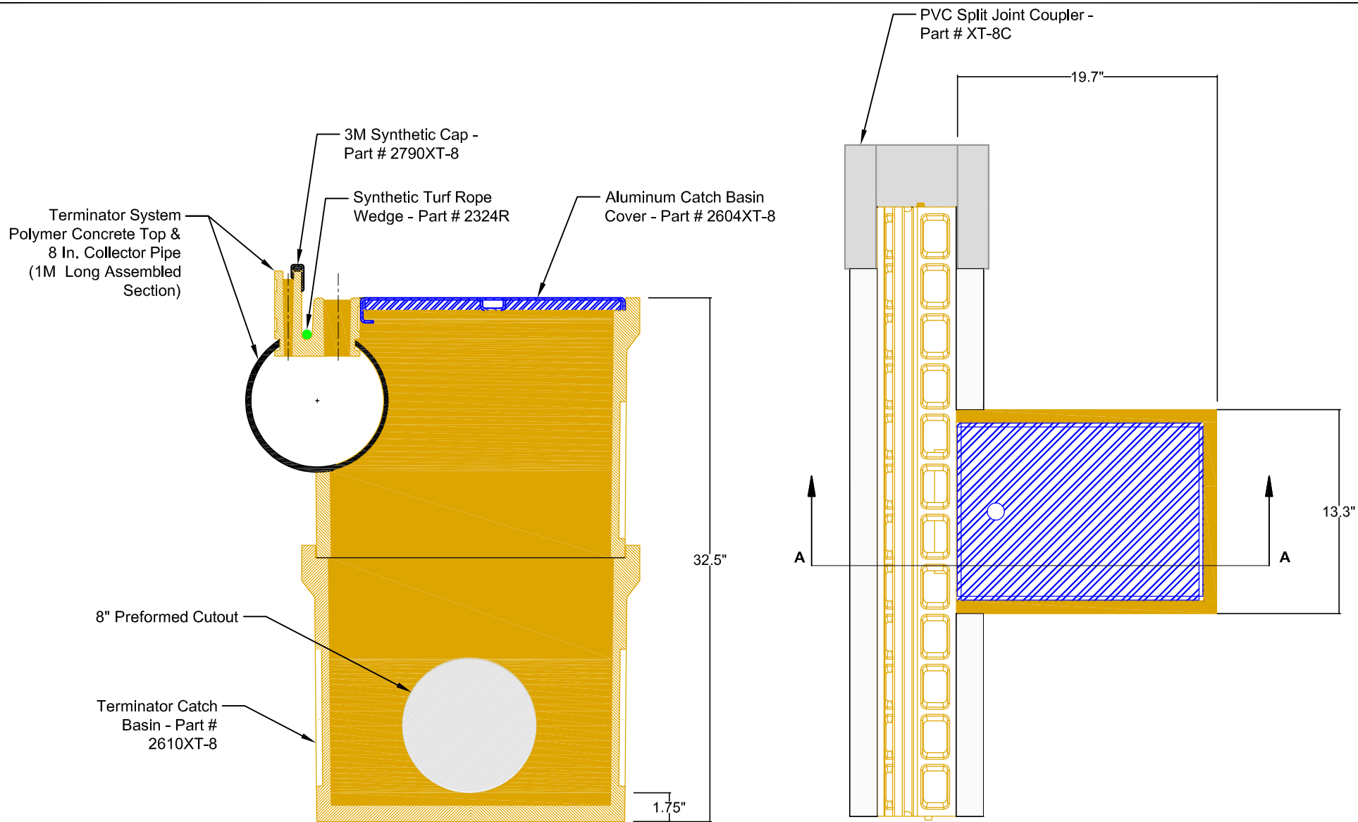
SECTION A-A
